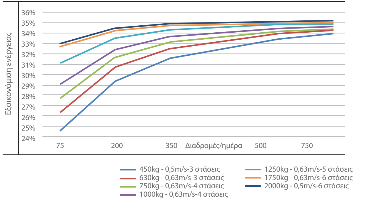
Εξοικονόμηση ενέργειας από τη χρήση VVVF (κατά ISO 25745-2)
