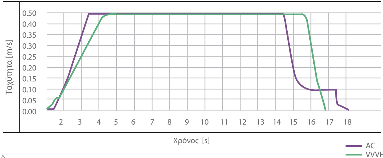
Διάγραμμα μεταβολής ταχύτητας
