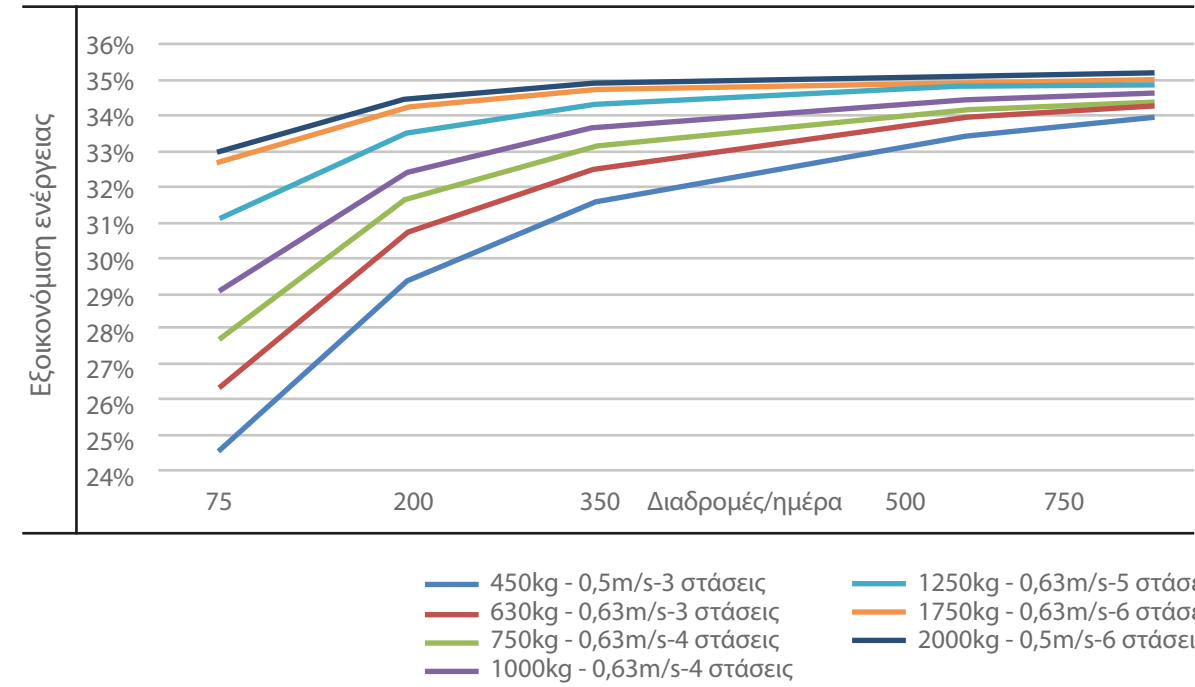
Εξοικονόμηση ενέργειας από τη χρήση VVVF (κατά ISO 25745-2)
